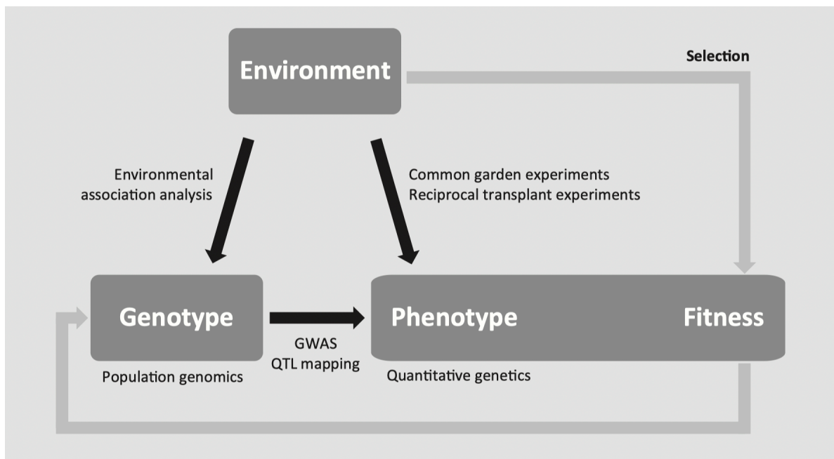
Figure 3: Rellstab et al 2015 (Image modified from Sork et al 2013)
